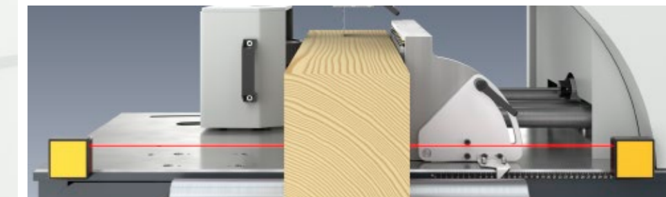
Automatische Breitenmessung des Werkstücks zur Positionierung der Vorschubrollen und des Breitenanschlags zur Steigerung der Produktivität
